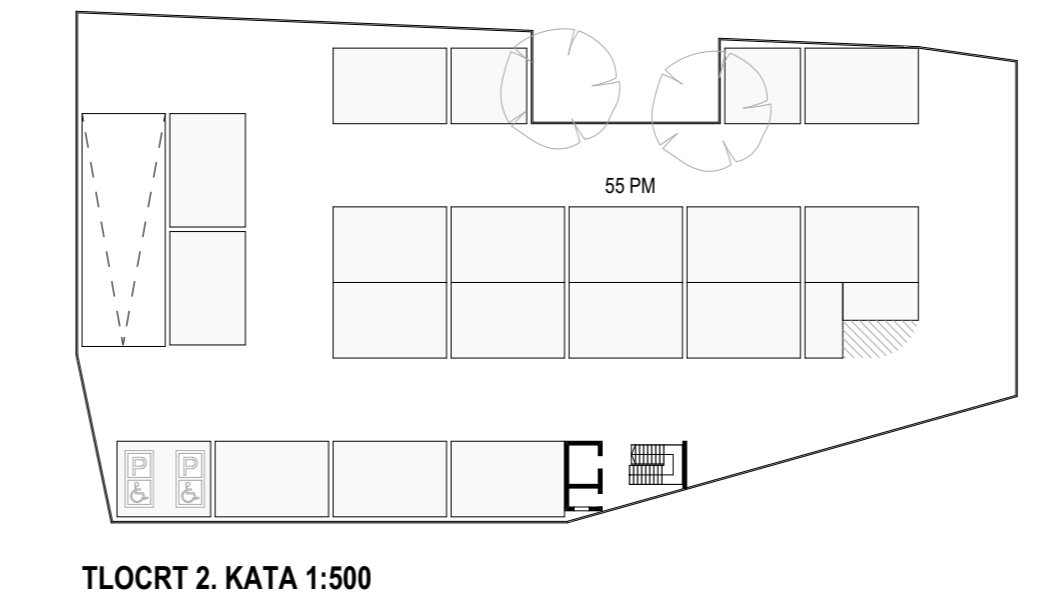
TLOCRT 2. KATA 1:500
