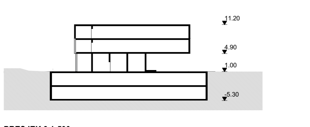
PRESJEK 3 1:500
