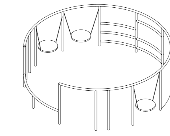
DJEČJE IGRALIŠTE - čelična konstrukcija sa ljuštarkama i mrežama za penjanje
