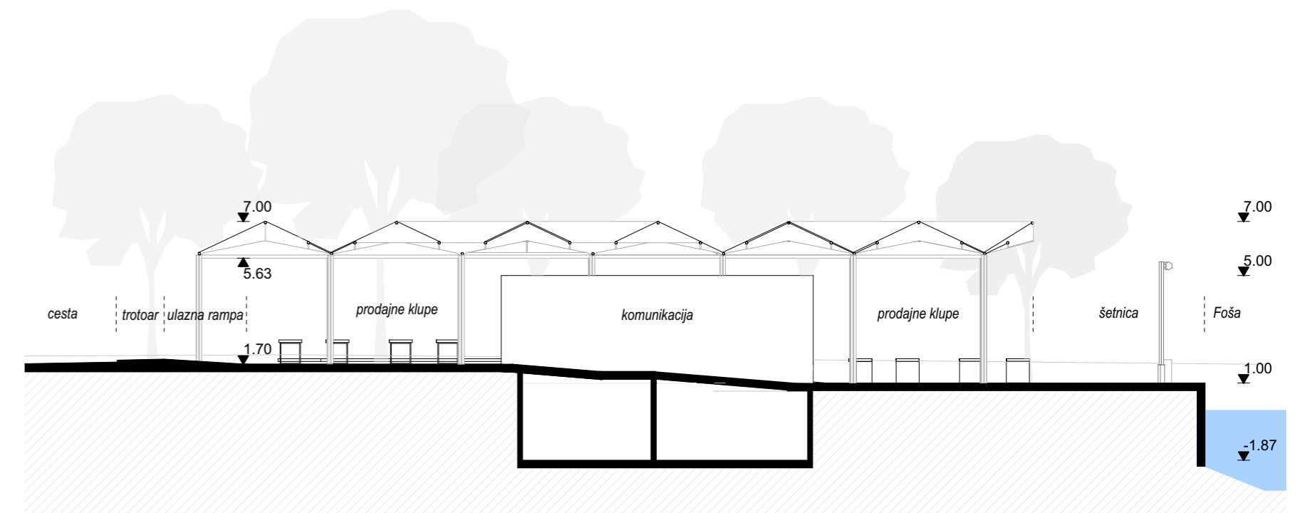
POPREČNI PRESJEK 1:200
