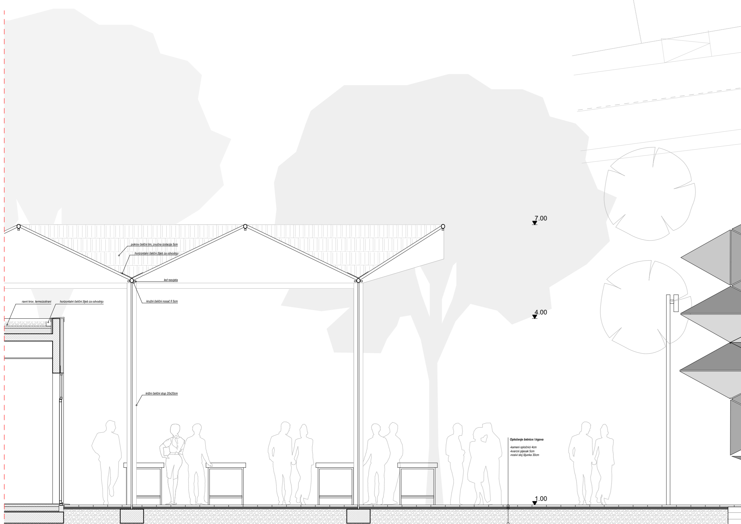
DETALJ 1:50
