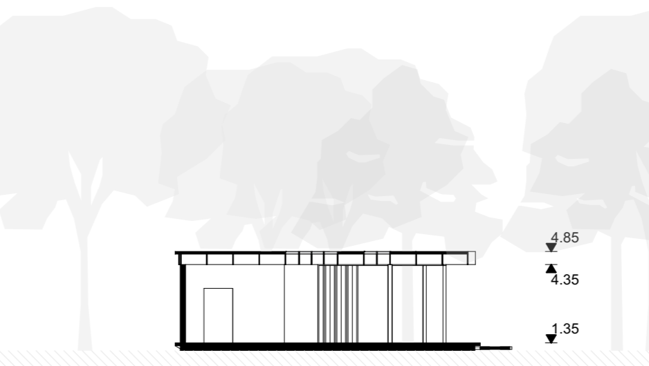
poprečni presjek 1:200
