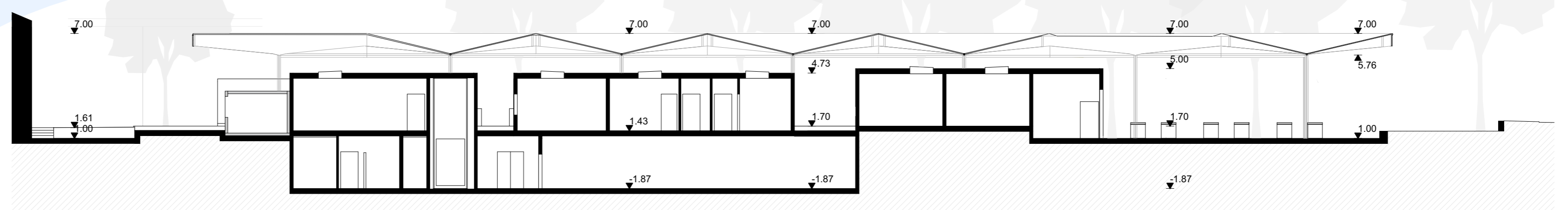
PODUŽNI PRESJEK 1:200
