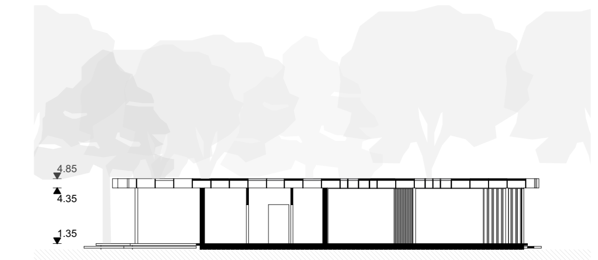
podni presjek 1:200
