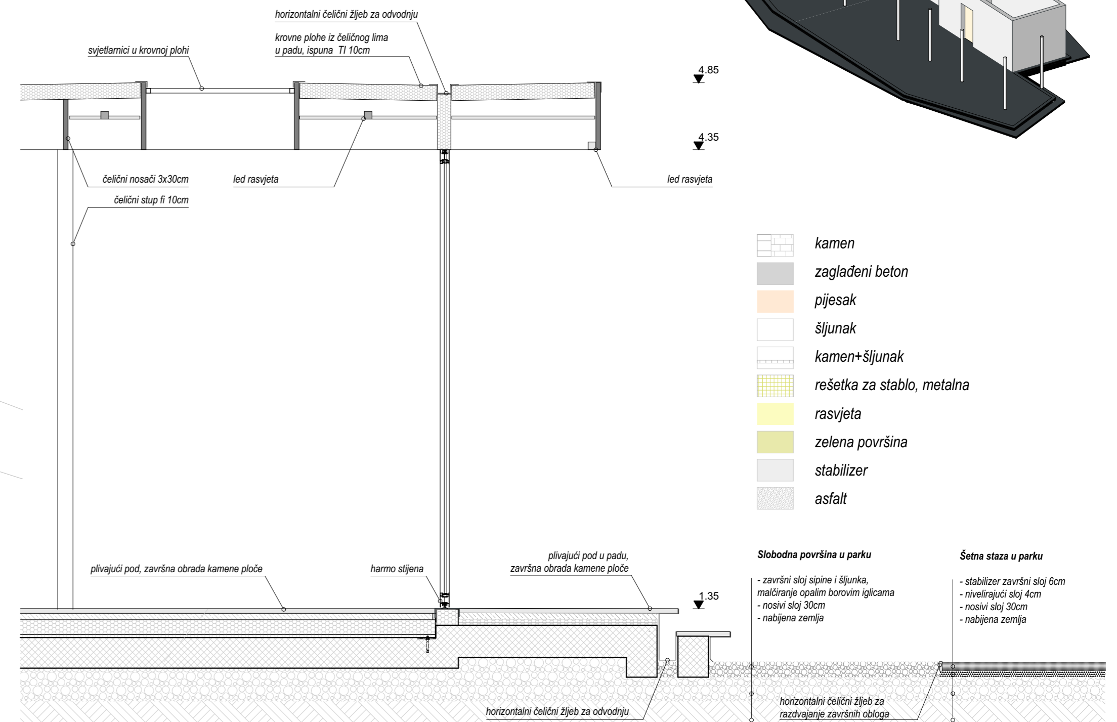
detalj 1:25
