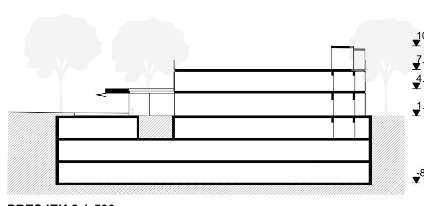
PRESJEK 2 1:500
